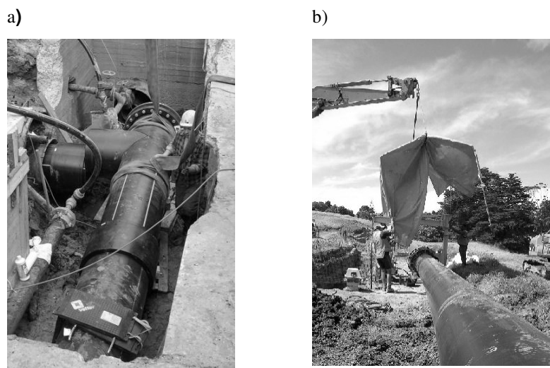
Rys.6. Przykłady wyrobów przeznaczonych do budowy dużych rurociągów i magistrali
