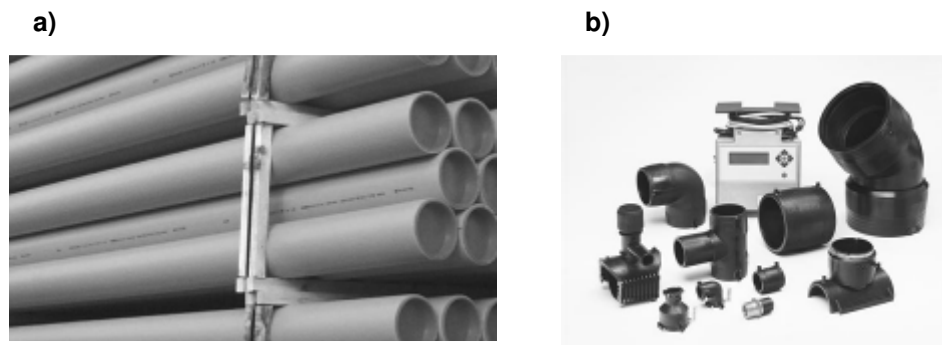
Rys.2. Przykłady wyrobów do budowy sieci przesyłania paliw gazowych: a) rury gazowe PE100 b) kształtki elektrooporowe
