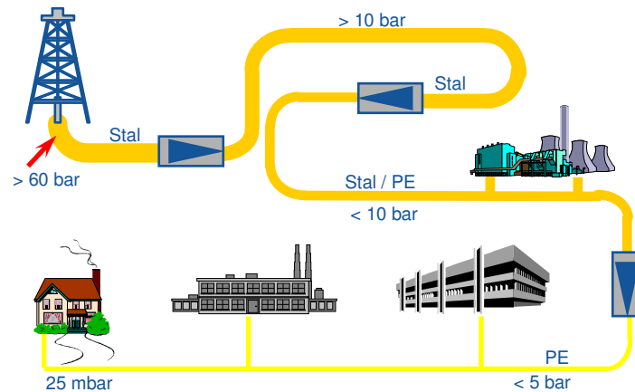
Rys.1. Schemat dystrybucji gazu
