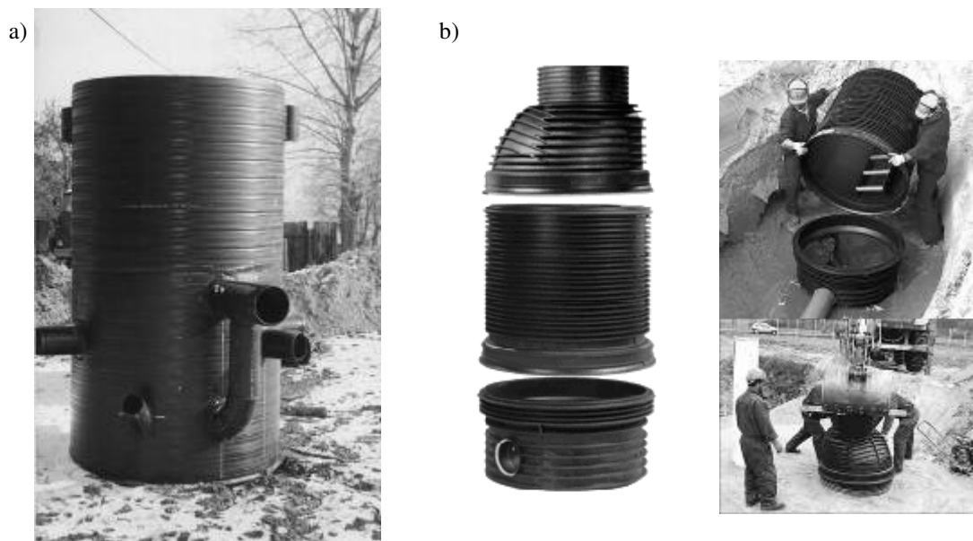
Rys.13. Przykłady studzienek z polietylenu: a) studzienka prefabrykowana Dn1200mm, b) studzienka modułowa Dn1000mm.
